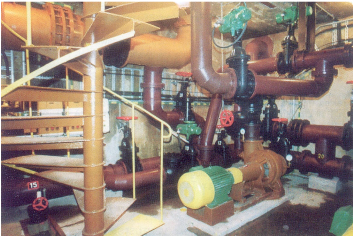
Maszynownia w prawym przyczółku jazu Zawada.
